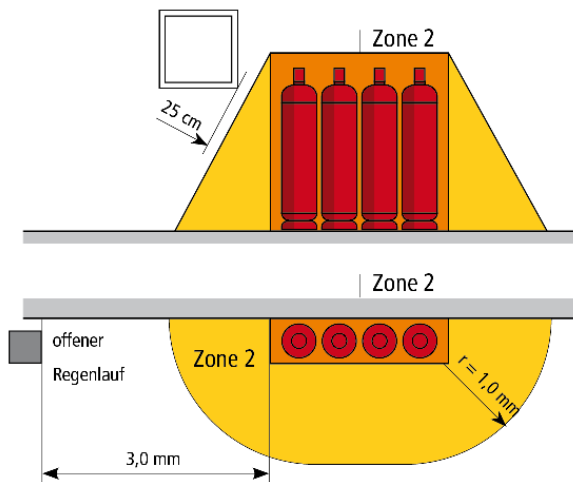
ExZonen Schrank
